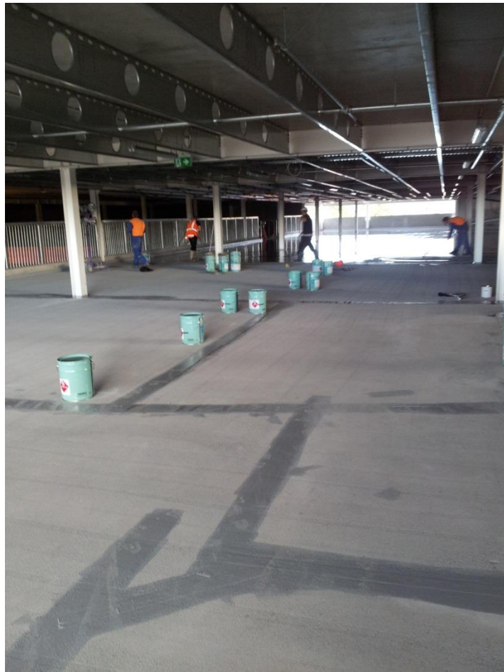
Membrane – Vulkem 350
